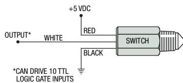
TTL Compatible Output
